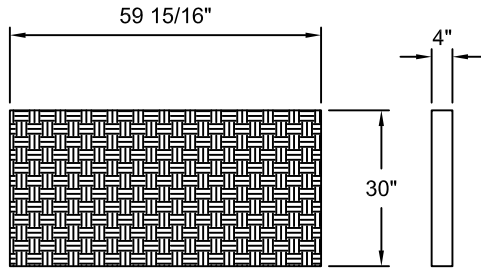
LHF30-60 SCALE: 1/2" = 1'-0" WEIGHT: 77#
