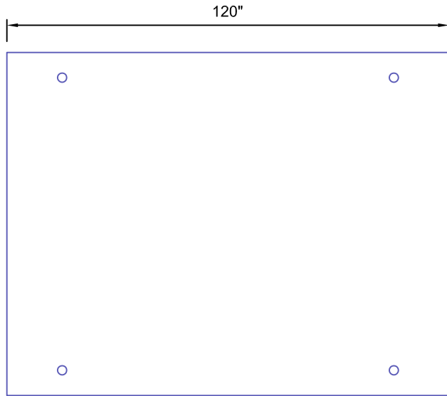
LHC8448-120 SCALE: 1/2"=1'-0"
