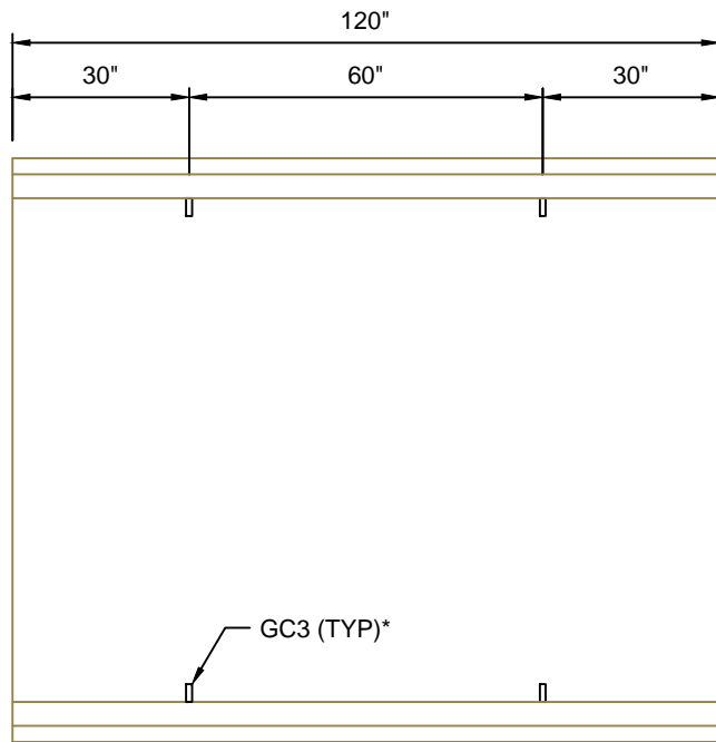
BHC8424-120 SCALE: 1/2"=1'-0"
