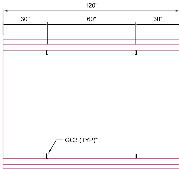
BHC7236-120 SCALE: 1/2"=1'-0"
