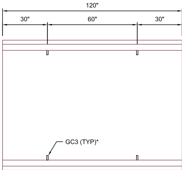
BHC7218-120 SCALE: 1/2"=1'-0"
