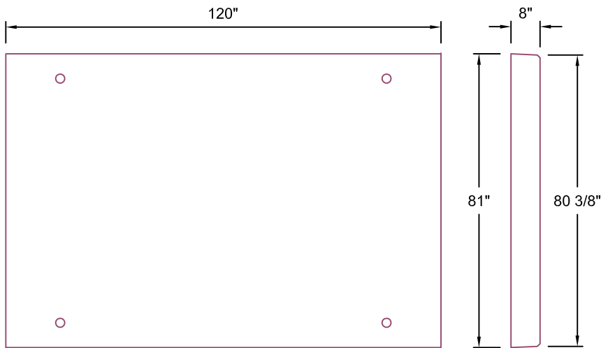
LHC7218-120 SCALE: 1/2"=1'-0"
