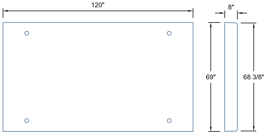
LHC6048-120 SCALE: 1/2"=1'-0"
