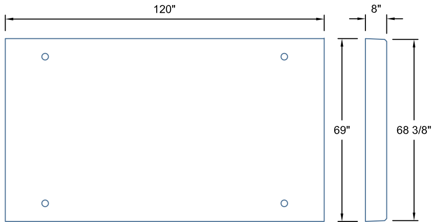
LHC6018-120 SCALE: 1/2"=1'-0"
