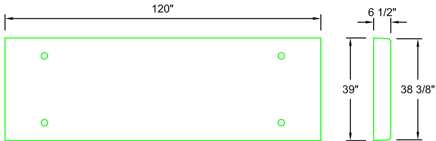
LHC3048-120 SCALE: 1/2"=1'-0"
