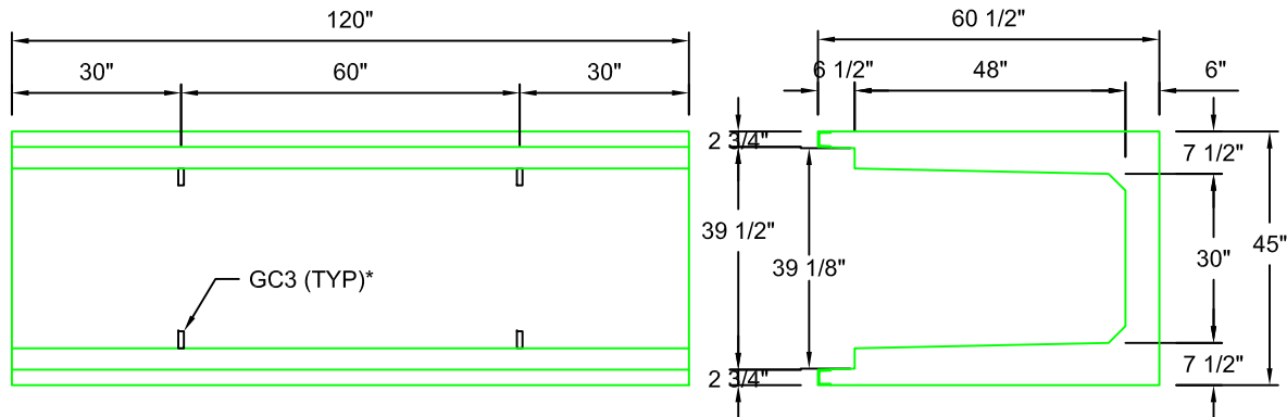
BHC3048-120 SCALE: 1/2"=1'-0"
