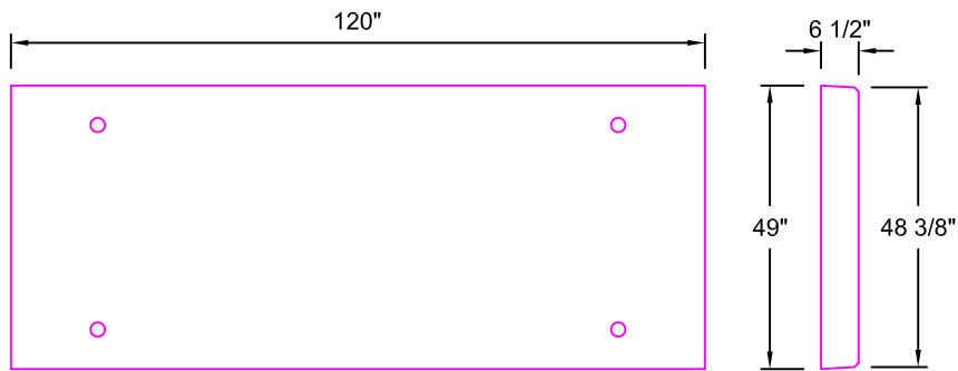
LHC4048-120 SCALE: 1/2"=1'-0"
