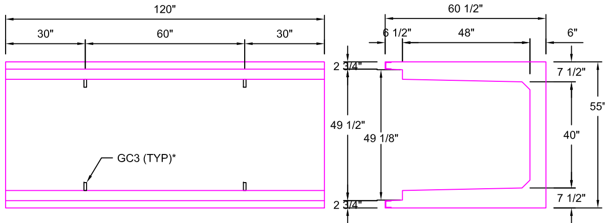
BHC4048-120 SCALE: 1/2"=1'-0"
