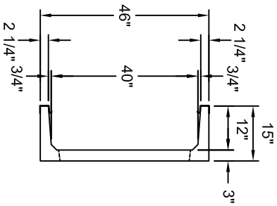
BP4012-120 SCALE: 1/2" = 1'-0"
